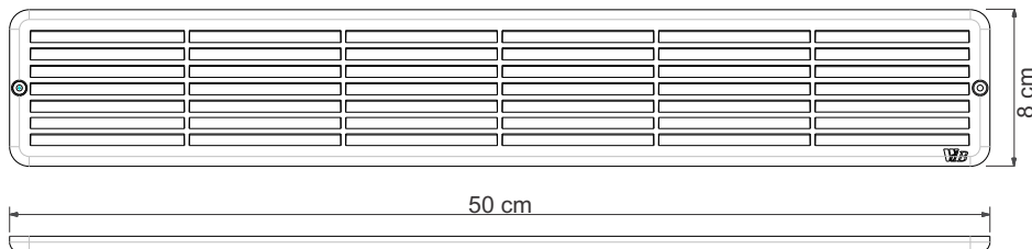
Desenho Técnico
