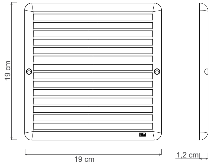
Desenho Técnico
